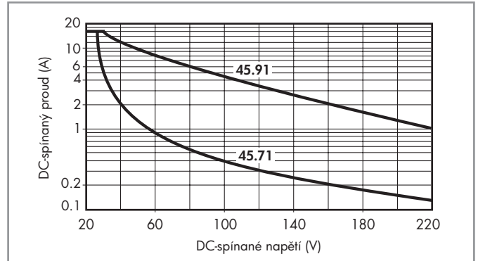
H 45 - spínací schopnost při DC1
